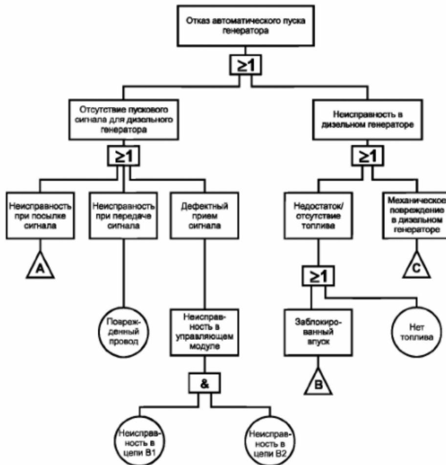
Рисунок А.1 – Пример «дерева неисправностей»
