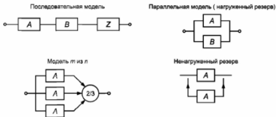
Рисунок A.5 — RBD для независимых блоков
