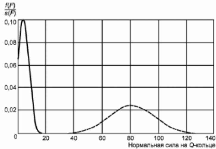
Рисунок А.12 — Пример применения критерия прочности напряжений
