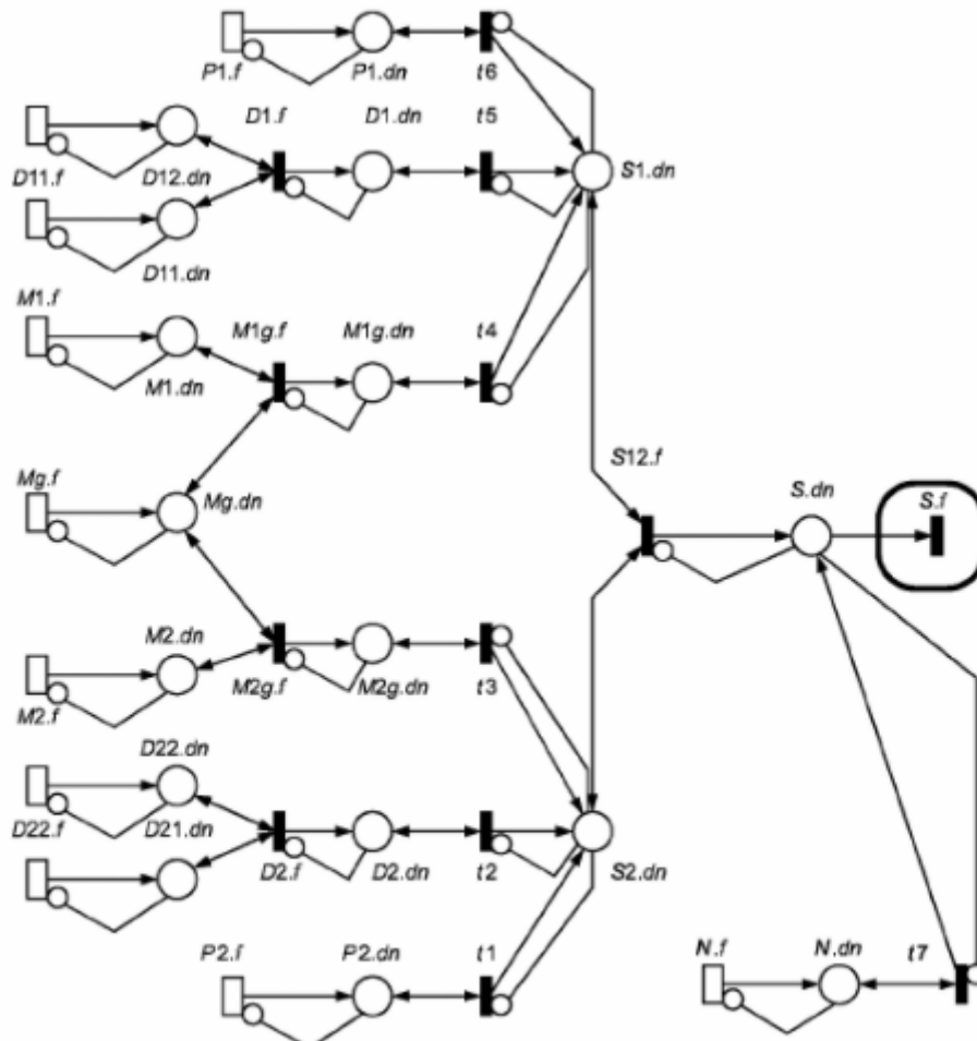
Рисунок А.9 — Сеть Петри мультипроцессорной системы
