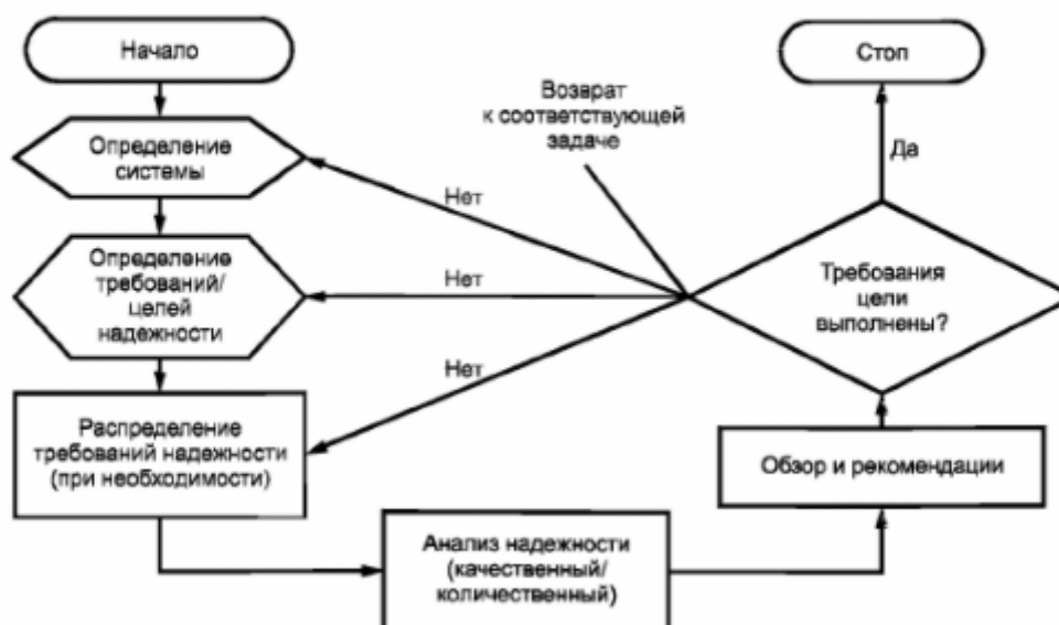
Рисунок 1 — Общая процедура анализа надежности
