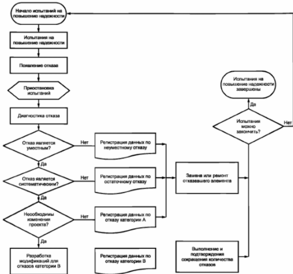
Рисунок 8 — Процесс испытаний на повышение надежности
